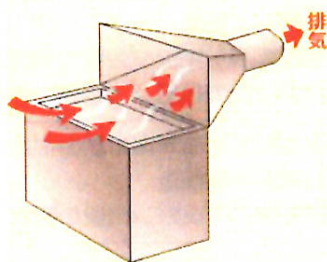
局所排気装置(外付け式)の例
